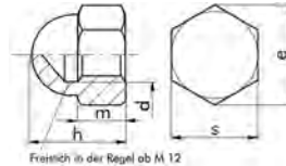
Freistich in der Regel ab M 12
